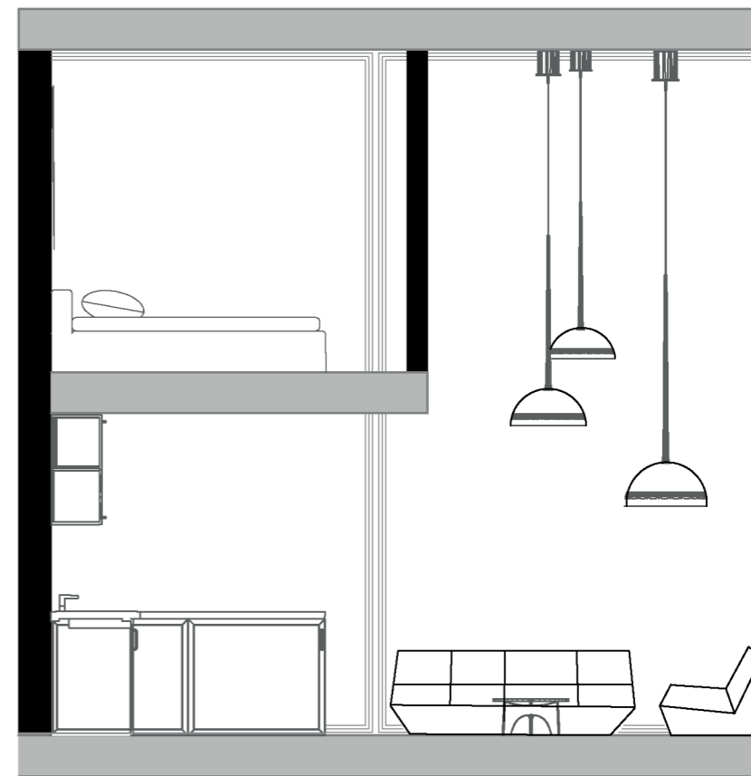
Przekrój B-B
