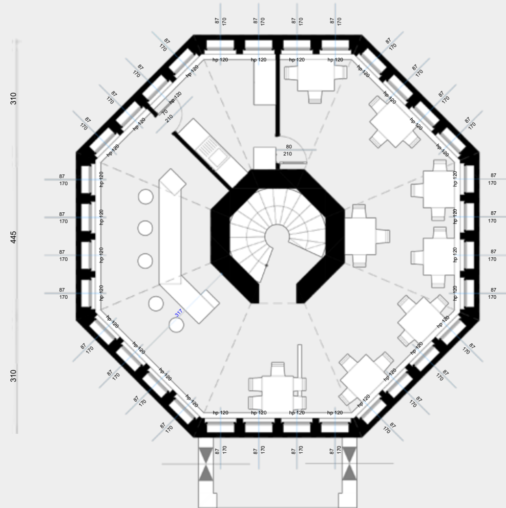
RZUT PIĘTRA
