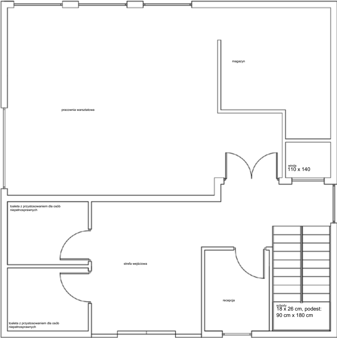
RZUT PARTERU:
