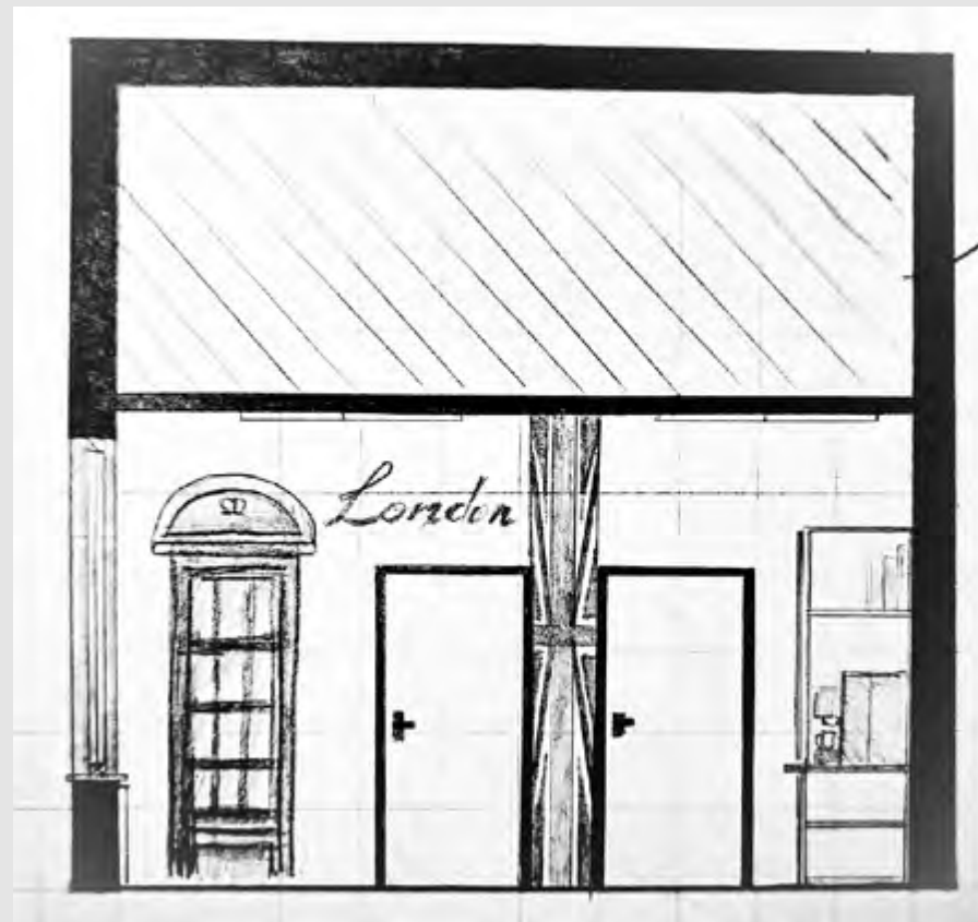
Przekrój boczny A
