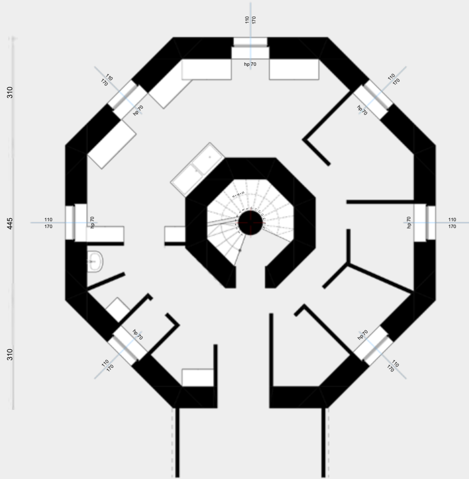
RZUT PRZYZIEMIA
