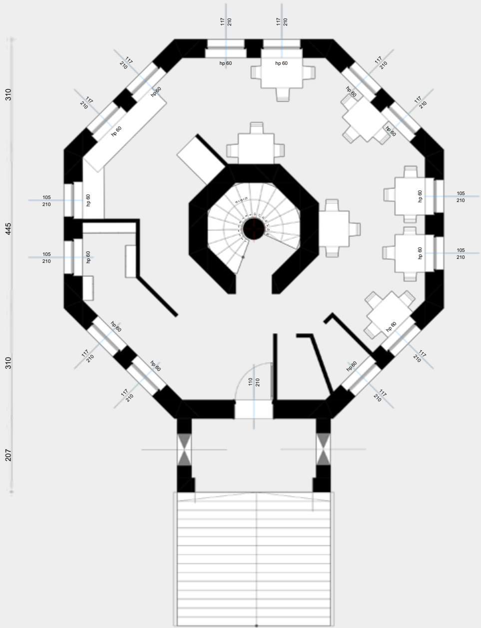
RZUT PARTERU
